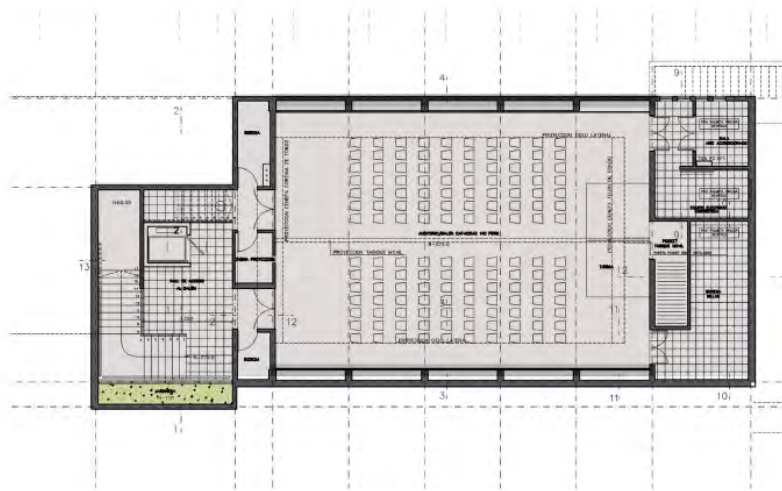
PLANTA NIVEL ACCESO
