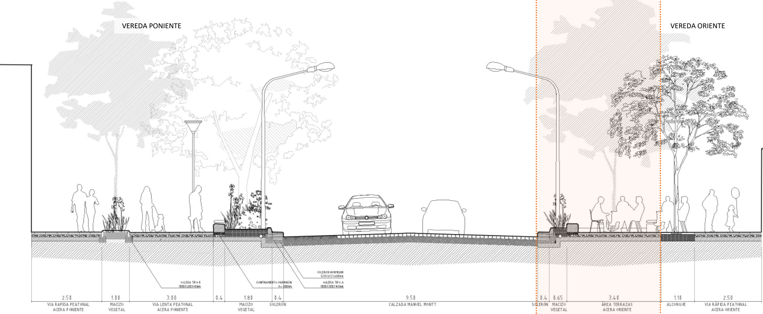
CORTE TIPO 02
